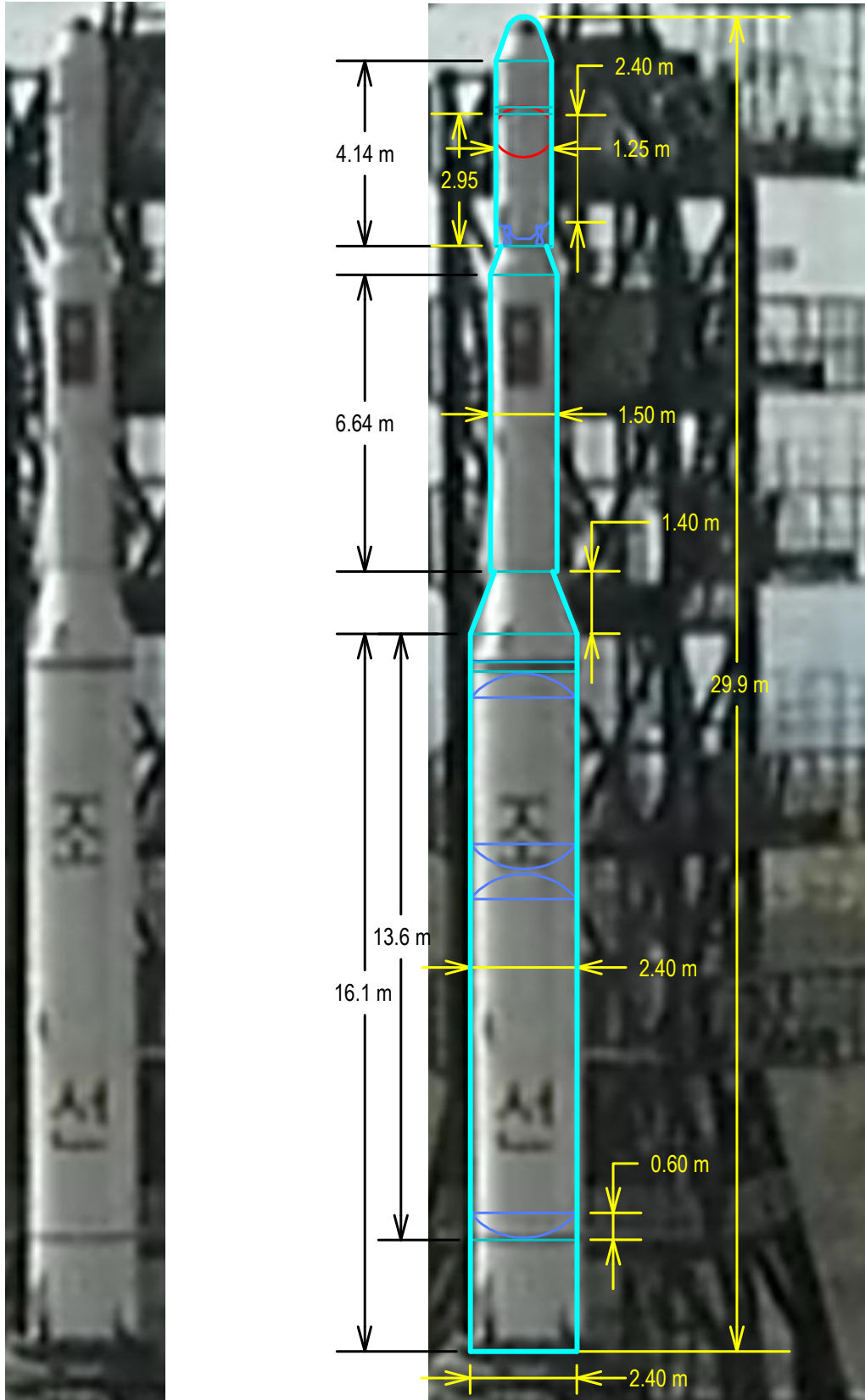
The Unha-2 Launcher (source T.A. Postol)
